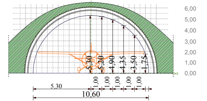
A HANGÁR KERESZTMETSZETE ÉS JELLEMZŐ FŐ MÉRETEI
