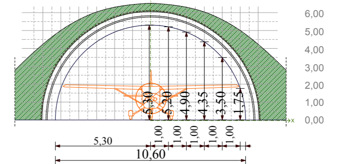
A HANGÁR KERESZTMETSZETE ÉS JELLEMZŐ FŐ MÉRTEI
